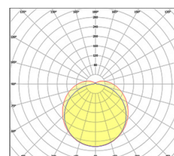
Röd kurva anger ljusspridningen tvärs armaturen
