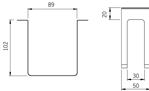
Väggfäste för släpljus upp / ned 1031684
